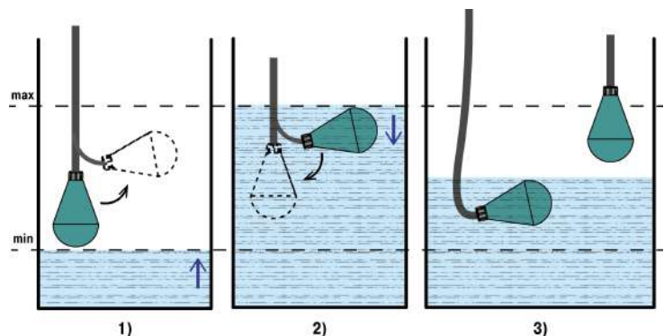
Рисунок 4.2 – Принцип действия
